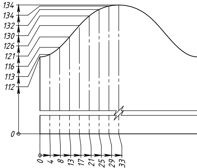
Поз.2 (Труба) развертка 1:1
